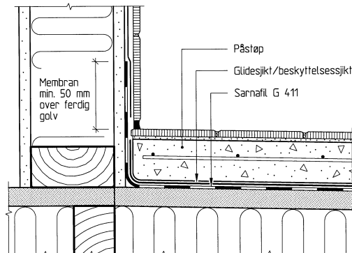
Fig. 5 Eksempel på anvendelse av Sarnafil G 411 i våtromsgolv
